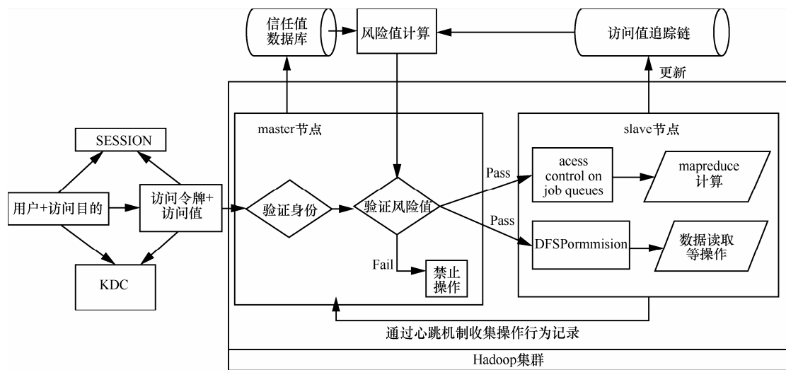
图 3 加入风险之后的 Hadoop 访问控制模型
