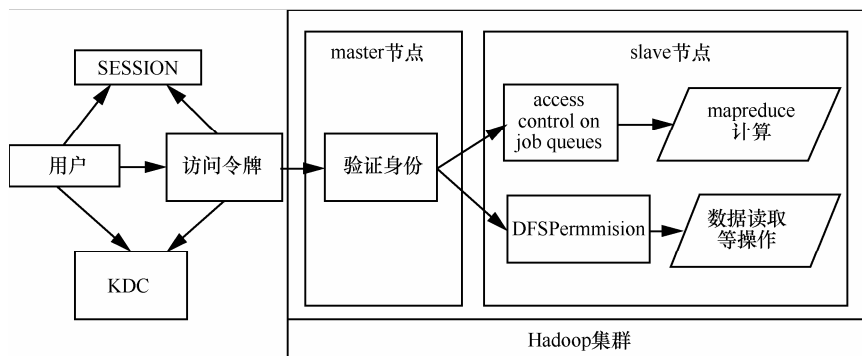
图 2 基于 Kerberos 的 Hadoop 访问控制模型
