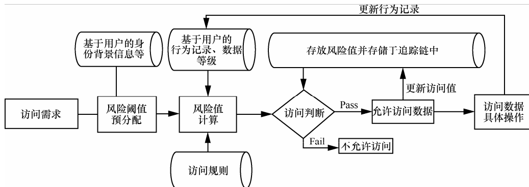
图 1 风险访问控制模型
